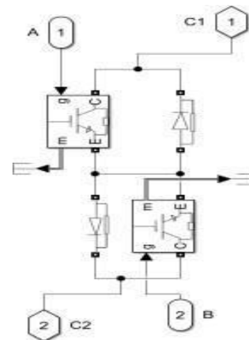
Rajah 7: Suis Penukar Matriks Dua Arah
