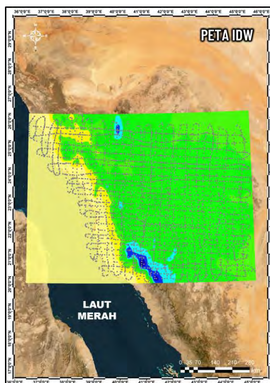
Rajah 10. Peta IDW
