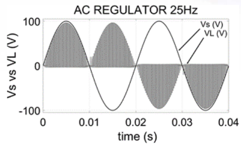
Rajah 19: Voltan Bekalan Dan Beban 25Hz
