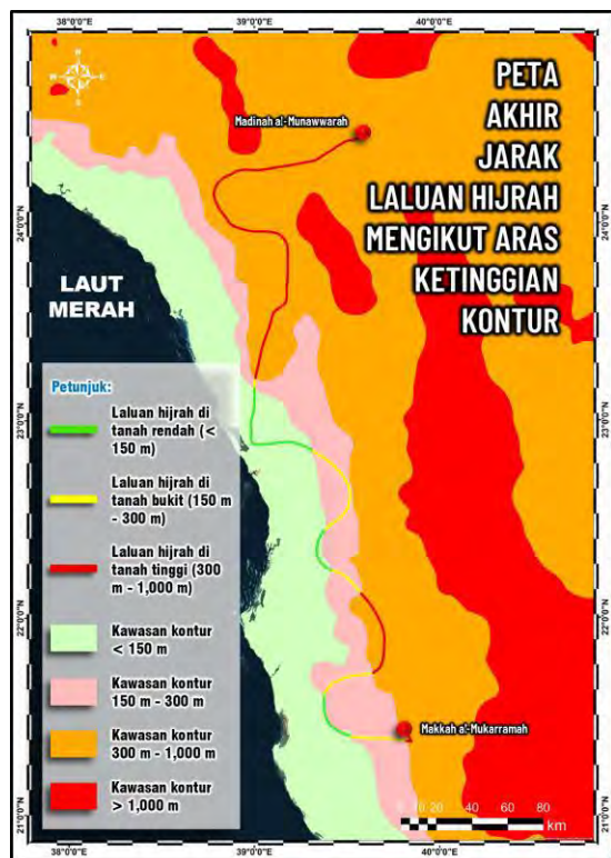
Rajah 16. Peta akhir menunjukkan jarak laluan hijrah mengikut aras ketinggian kontur
